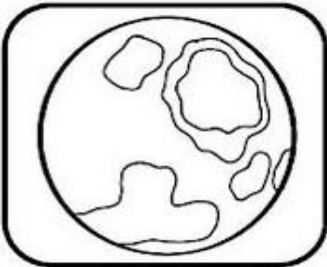
MARTE
