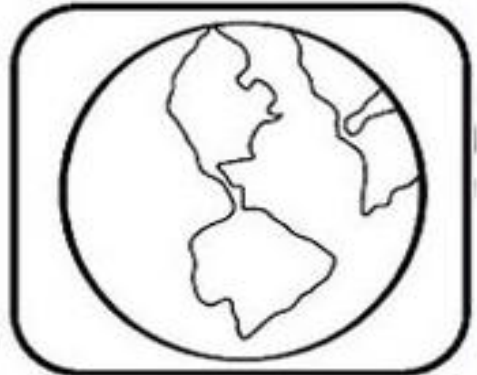
TIERRA
