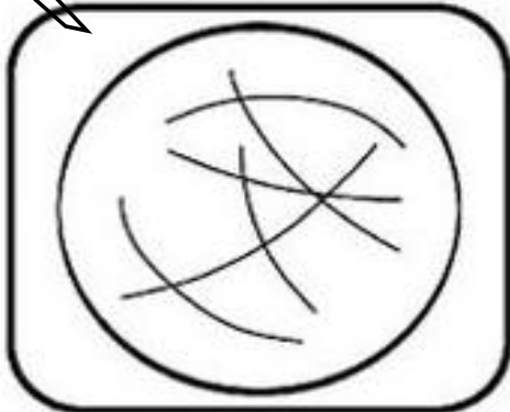
MERCURIO
