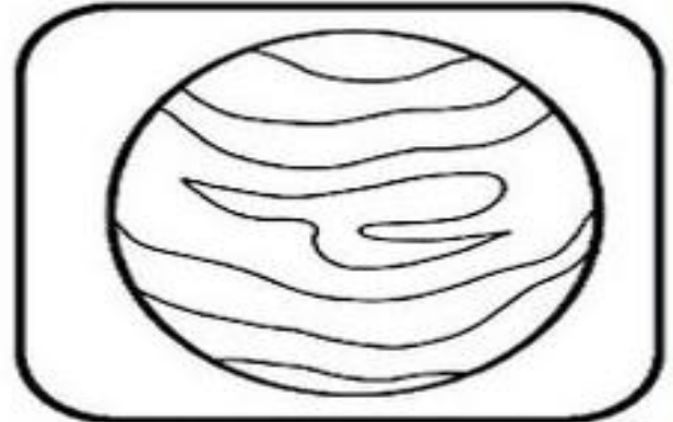
NEPTUNO
