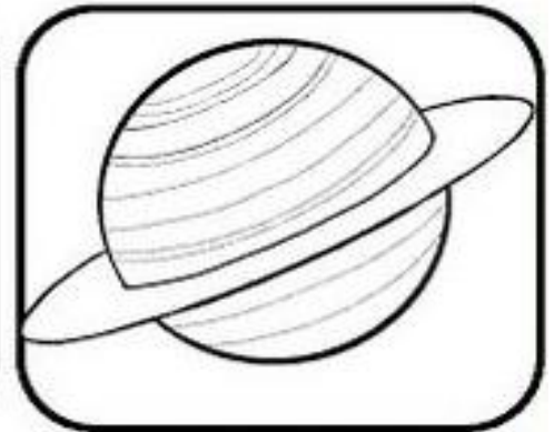
SATURNO
