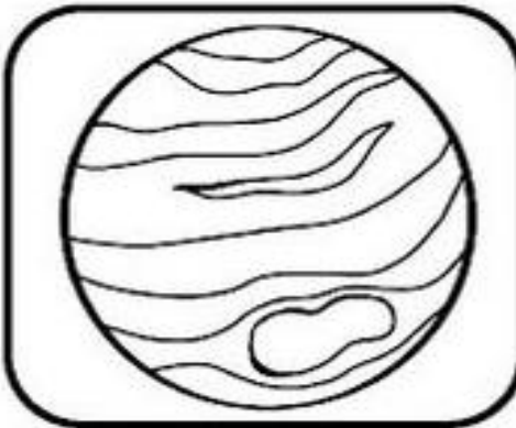
JÚPITER
