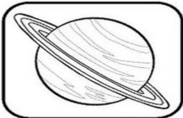
URANO
